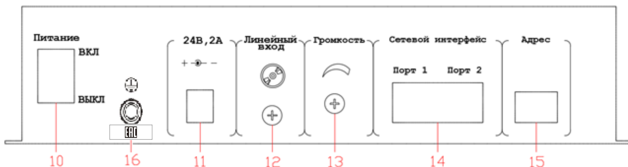
Рис. 2.2. LPA-DUO-MIC (задняя панель)
